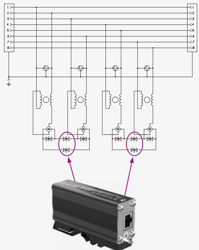
obr. 3 Univerzální ochrana pro jednu linku Ethernet s PoE – DL-xG-RJ45-PoE-AB (zvýrazněny ochranné prvky PoE)
