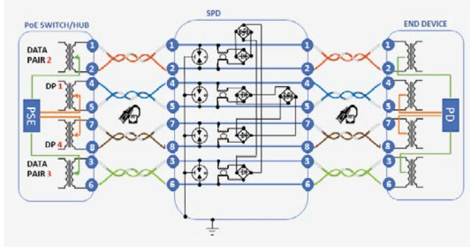
obr. 4 Schéma ochrany Ethernet linky s PoE pomocí DL-xG-RJ45-PoE-AB
