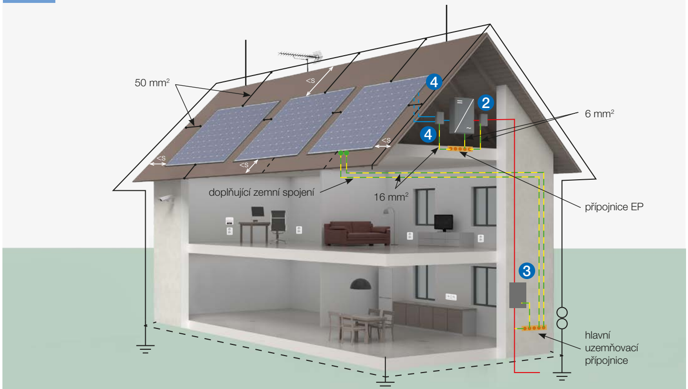
obr. 5 Nedodržená přeskoková vzdálenost „s“ mezi FVE panely a hromosvodnou soustavou
