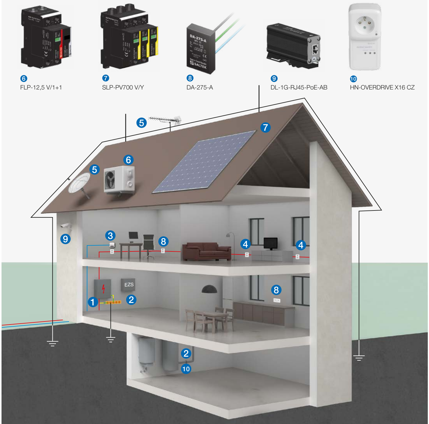
obr. 1 Příklad instalace přepětových ochran v rodinném domě
