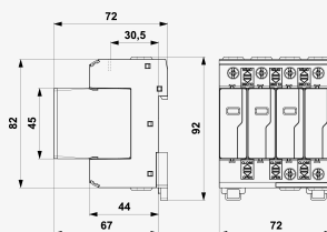
Rozmery produktu
