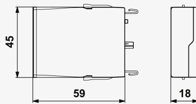
Rozmery produktu
