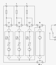
Schéma zapojenia
