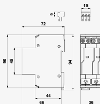
Rozmery produktu
