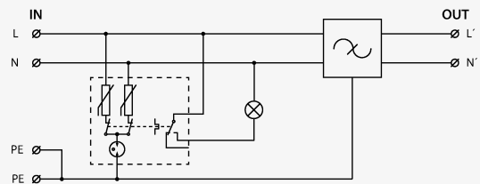
Schéma zapojenia
