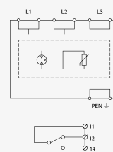
Schéma zapojenia
