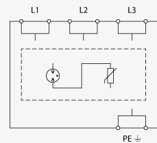
Schéma zapojenia
