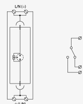
Schéma zapojenia
