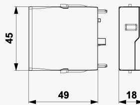
Rozmery produktu
