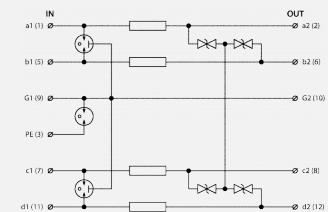
Schéma zapojenia
