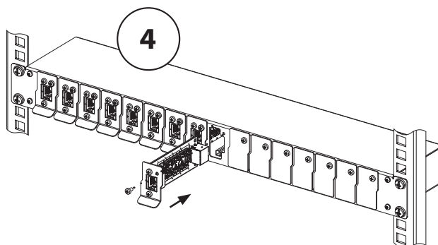
Orientace přepětových ochran (IN/OUT) musí být shodná. / The orientation of the surge protective devices (IN/OUT) must be the same.
