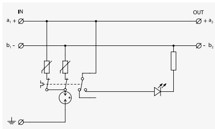
DMP-024-V/1-JFR1 (see Fig. 38)
