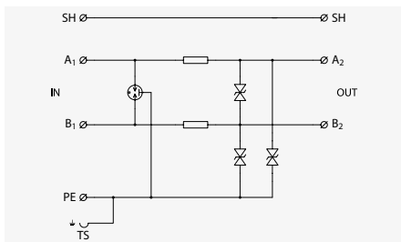
BDM-012-V/2-FR1 (see Fig. 44)
