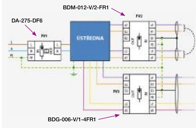
obr. 49 Ochrana komunikace IB 2
