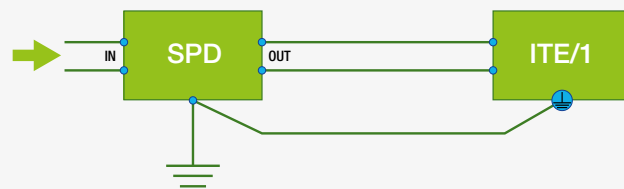
obr. 17 Správné připojení ochranné země
