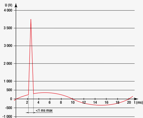
obr. 1 Přechodné přepětí
