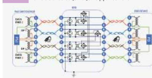
obr. 54 PoE dle standardů „at“ a „bt“ a jejich ochrana
