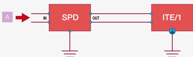
obr. 16 Chybné připojení ochranné země
