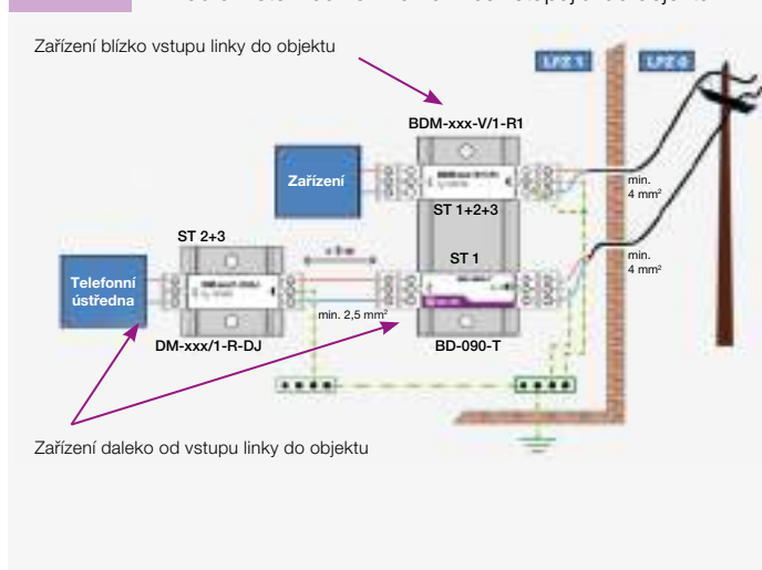
obr. 11 Příklad umístění ochran na na lince vstupující do objektu
