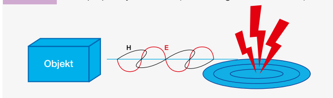
obr. 7 Šíření přepětí vyzařováním (elektromagnetickou vazbou)
