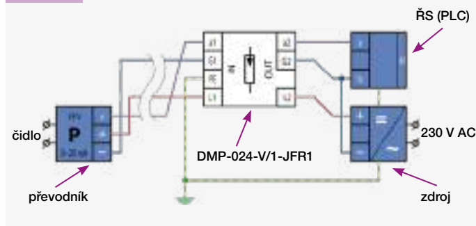
obr. 38 S externím napájením – společný vodič
