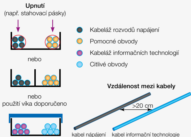
obr. 13 Možné uložení svazků
