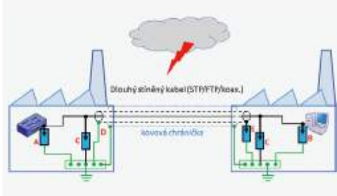
obr. 55 Zemnění dlouhého stíněného kabelu / svazku / kabelovodu / žlabu
