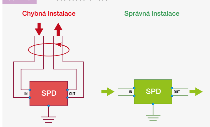
obr. 14a Eliminace souběhů vedení
