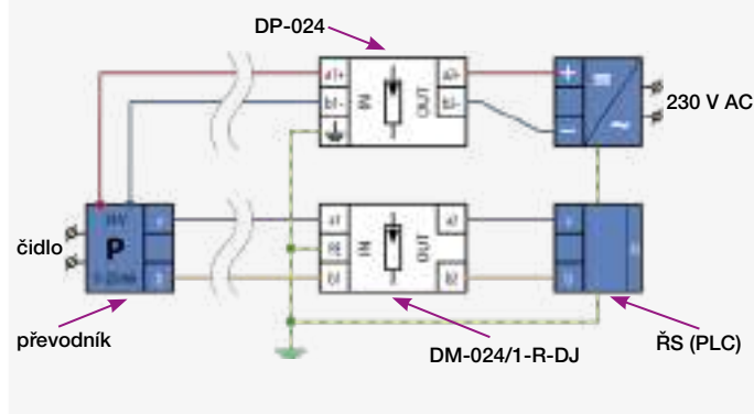
obr. 37 S externím napájením
