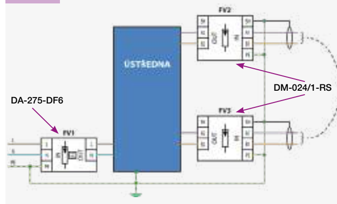
obr. 43a Varianta pro proud do 500 mA
