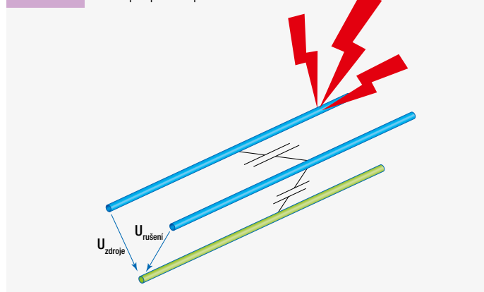
obr. 6a Šíření přepětí kapacitní vazbou
