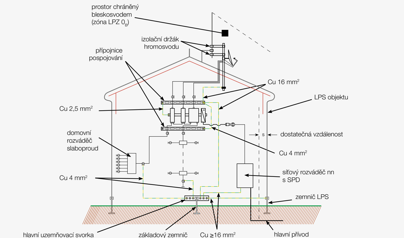
obr. 2 Instalace doplňkového izolovaného jímáče pro ochranu anténních systémů. (viz norma EN 60728-11 ed.3, obr. 12)
