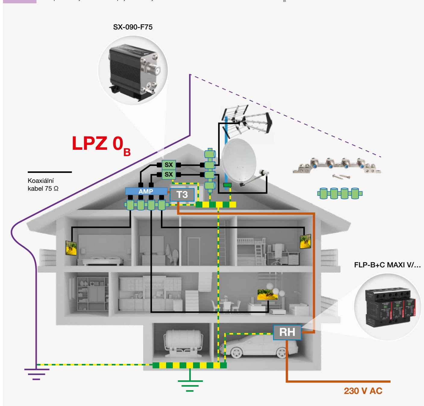
obr. 5 Princip ochrany komerčních přijímacích systémů R/TV/SAT s anténou umístěnou v LPZ 0 p .
