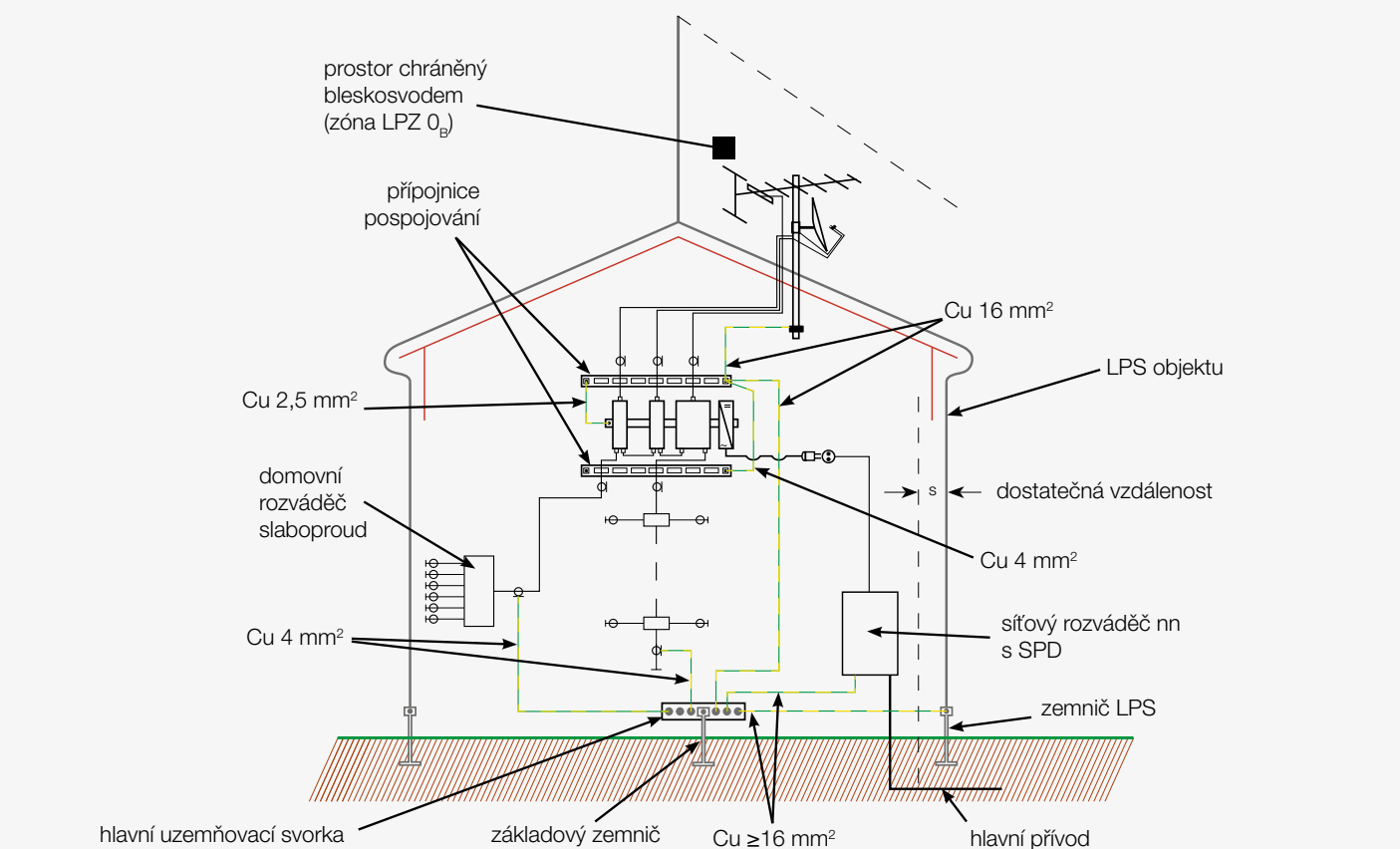
obr. 1 Instalace anténních systémů do prostoru LPZ 0 B . (viz norma EN 60728-11 ed.3, obr. 11)
