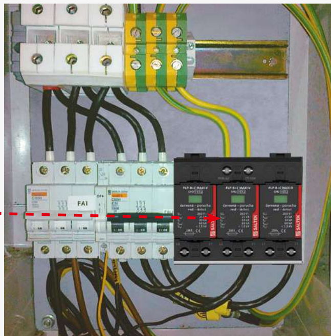
Správně: přetočením SPD (obr. 13 b) se zpřehlední zapojení v rozvaděči a zároveň se splňuje podmínka z ČSN 33 2000-5-534 ohledně smyček.
