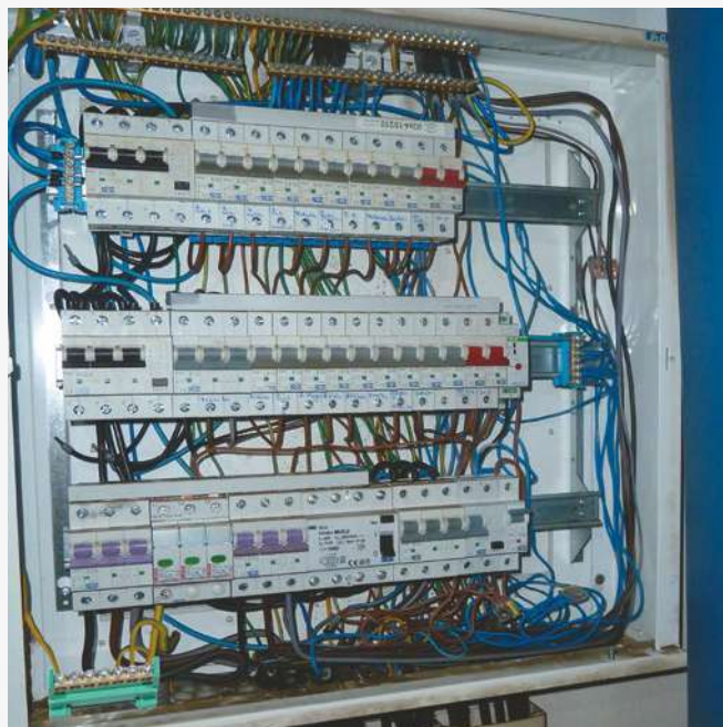
Chybně: montáž SPD nesplňuje podmínky ČSN 33 2000-5-534 – délka připojovacích vodičů.
