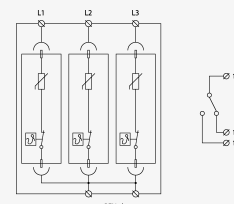
Prinzipschaltbild
