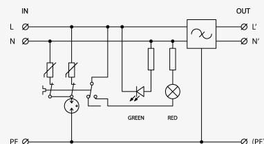
Prinzipschaltbild
