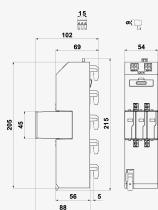
Produktabmessungen
