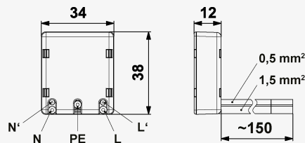
Produktabmessungen
