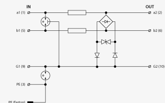
Prinzipschaltbild
