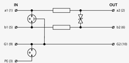
Prinzipschaltbild
