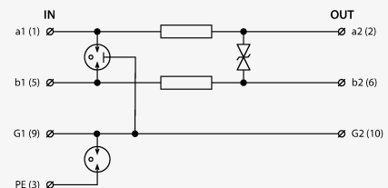
Prinzipschaltbild
