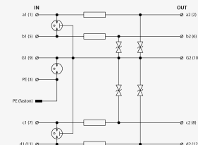
Prinzipschaltbild
