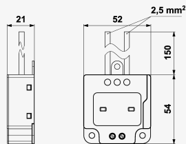
Produktabmessungen
