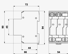
Produktabmessungen
