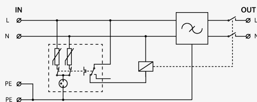
Prinzipschaltbild
