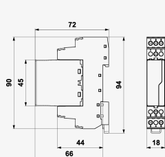
Produktabmessungen
