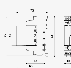
Produktabmessungen
