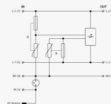
Prinzipschaltbild
