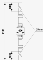
Produktabmessungen
