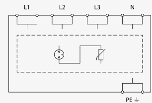
Prinzipschaltbild
