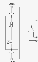
Prinzipschaltbild
