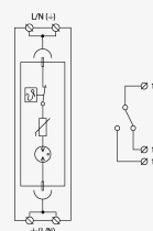
Prinzipschaltbild
