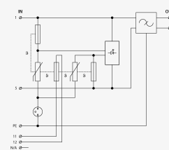
Schéma zapojení
