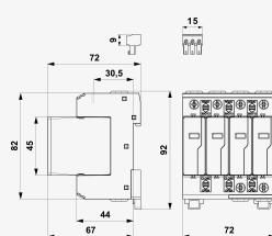
Rozměry
