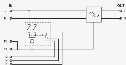
Schéma zapojení
