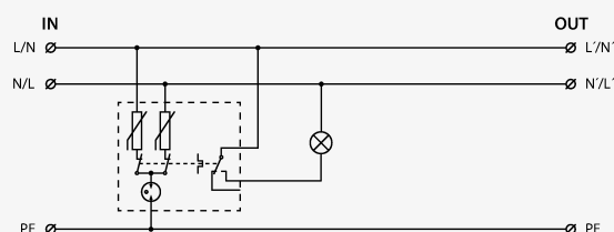
Schéma zapojení
