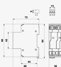
Rozměry
