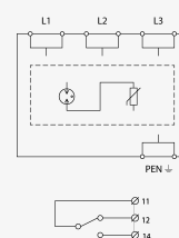
Schéma zapojení
